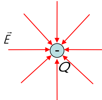
Pole elektryczne od ujemnego ładunku punkowego
